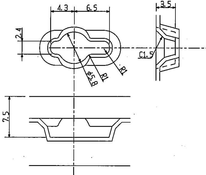
Detail A (5:1) 詳細 A (5:1)
